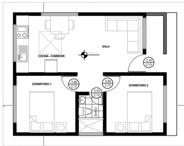
PLANTA ARQUITECTÓNICA VIVIENDA SOCIAL ESC. GRÁFICA
