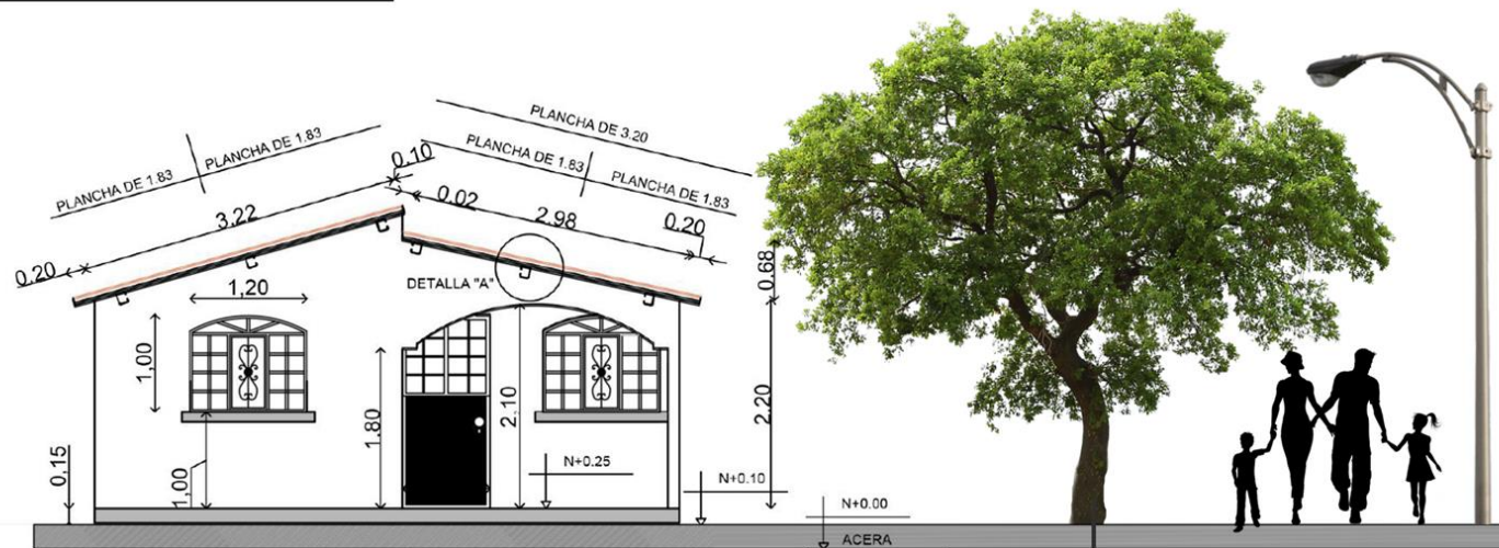
FACHADA FRONTAL ESC. GRÁFICA
