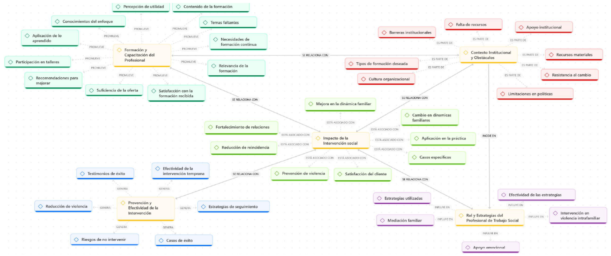
Figura 1 Red Semántica
