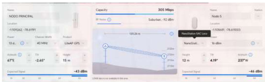
Figura 39. Simulación del enlace NP-N5 en UISP Design Center
