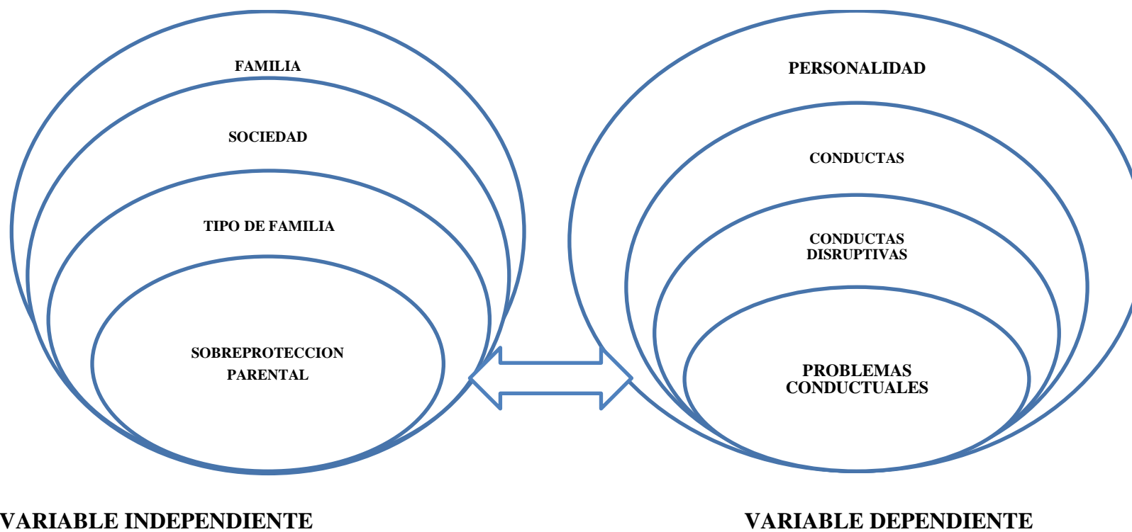
Gráfico N° 2 Categorías Fundamentales
