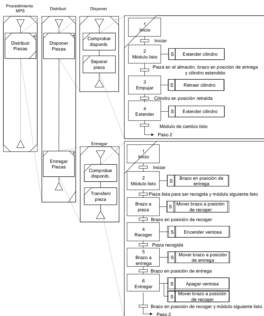
Figura 11. Ejemplo de procedimiento de receta de control de la estación de distribución
