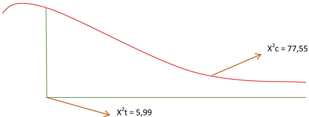
Gráfico No. 13 Campana de Gauss
