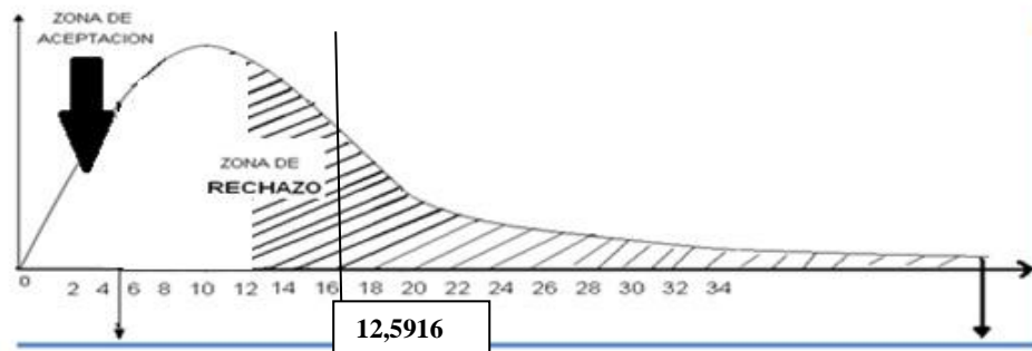
Gráfico N° 25 Representación Gráfica Chi – Cuadrado T
