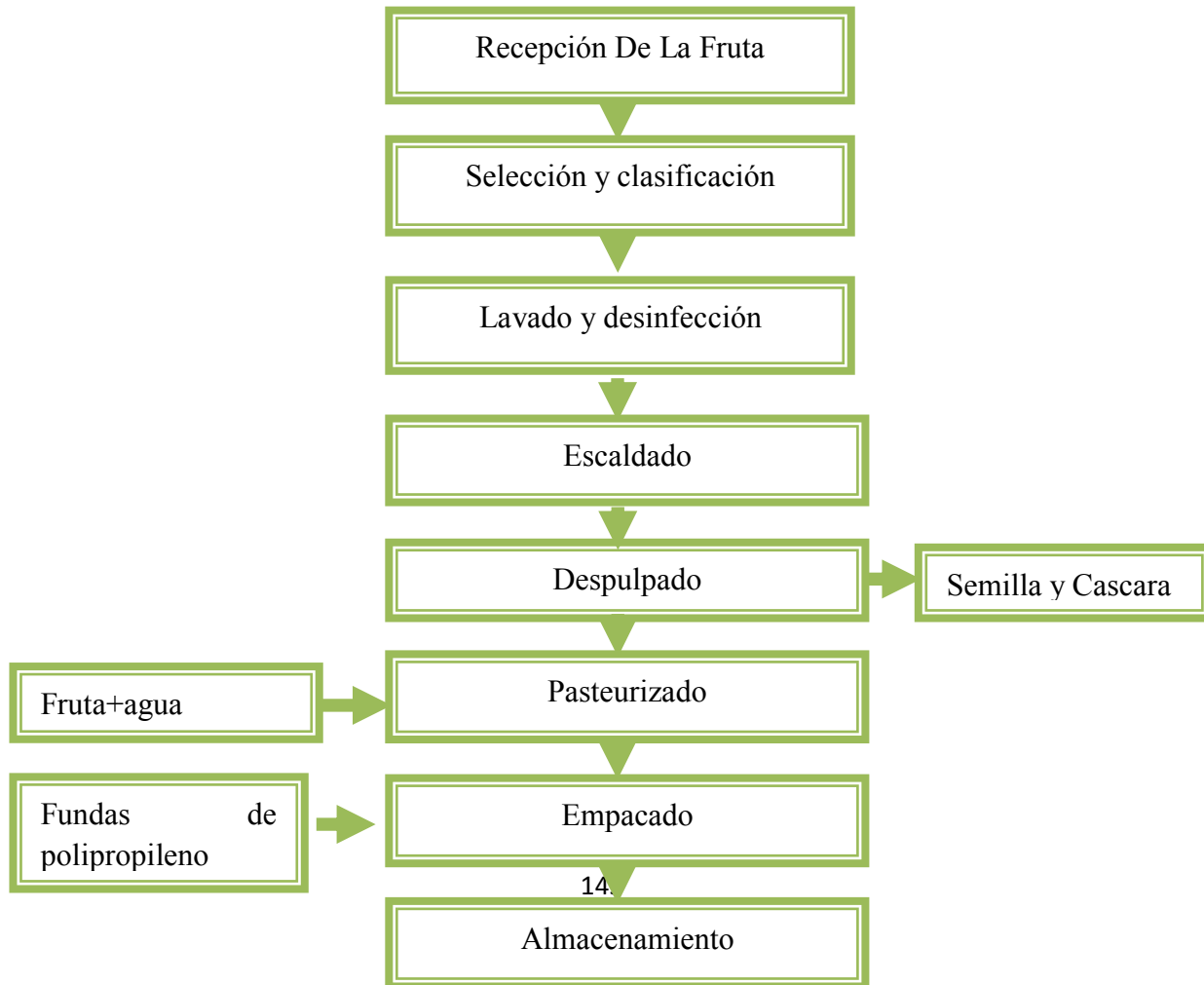
Gráfico N°. 45. Diagrama de proceso de elaboración
