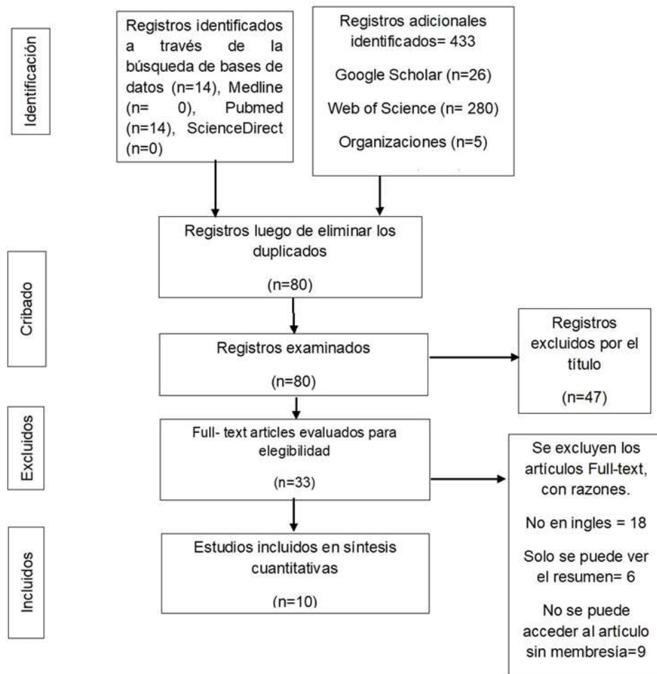
Figura 1. Flujograma PRISMA
