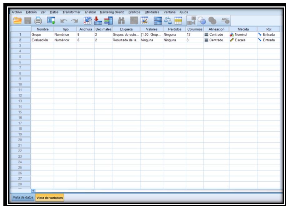
GRÁFICO 14: Supuesto normalidad
