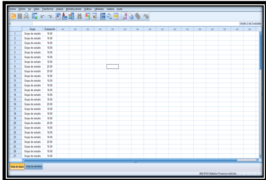
Gráfico 15: Ingresar datos:
