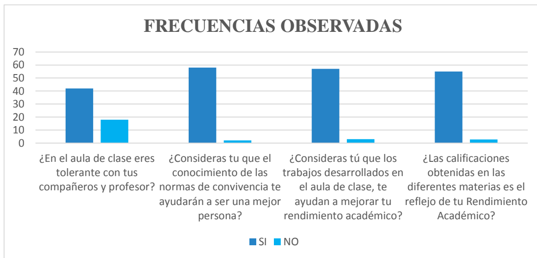
Gráfico N° 30: Frecuencias Observadas
