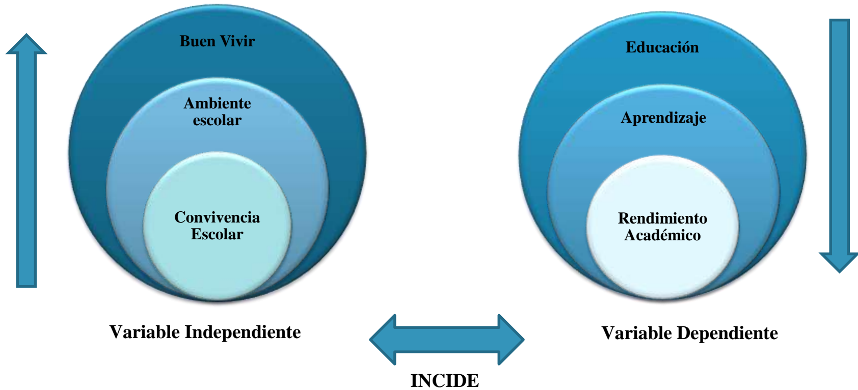
Gráfico N° 2: Análisis Categorial
