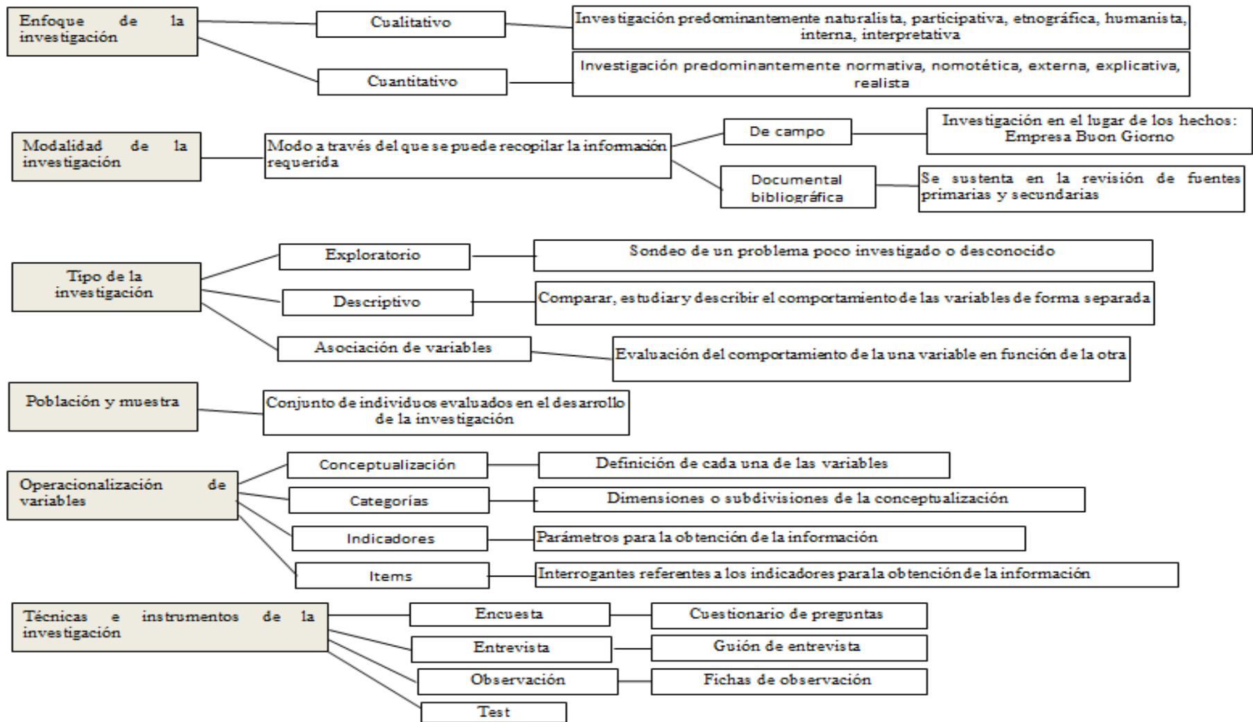
Ilustración 6: Etapa 3: Metodología
