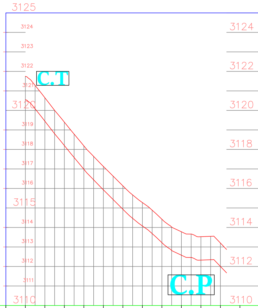
calle 2 -0+010.00 - 0+120.00
