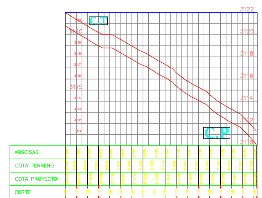
Calle 20 0+000.00 - 0+173.00
