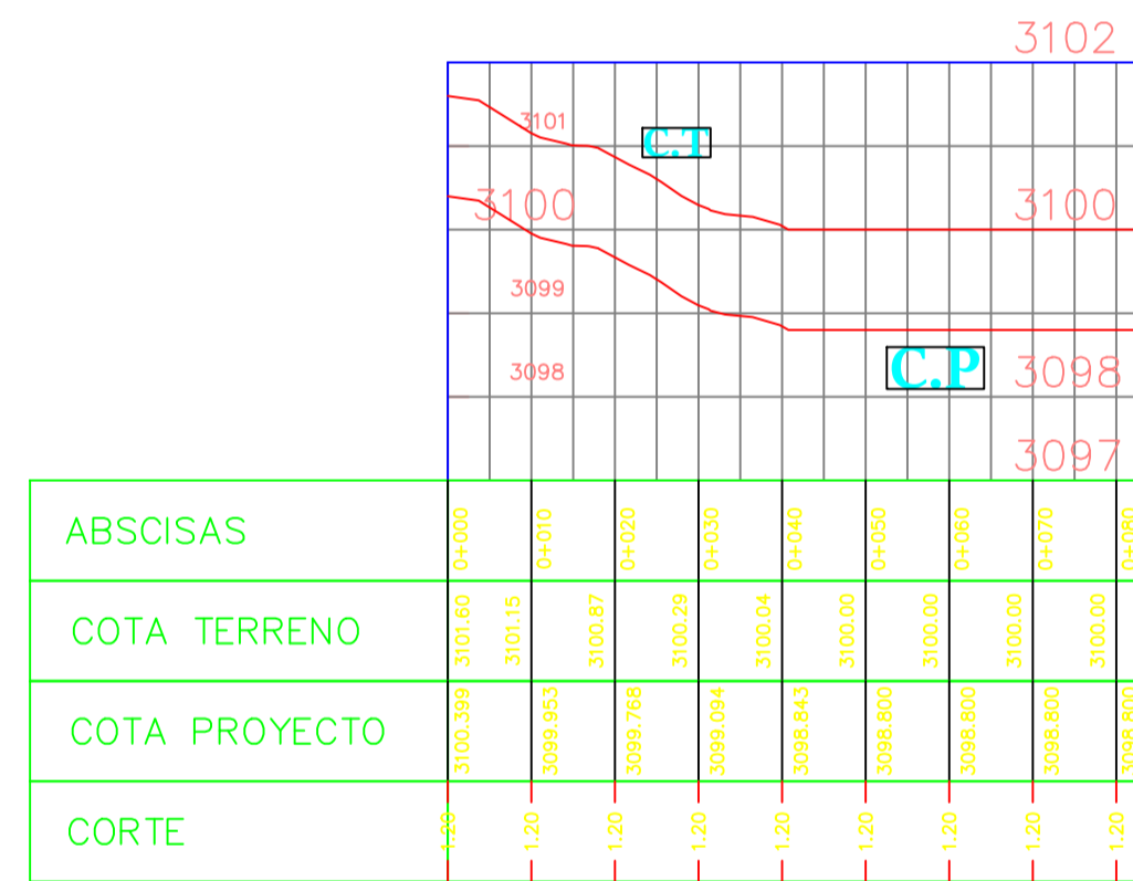
Calle 18 0+000.00 - 0+083.00
