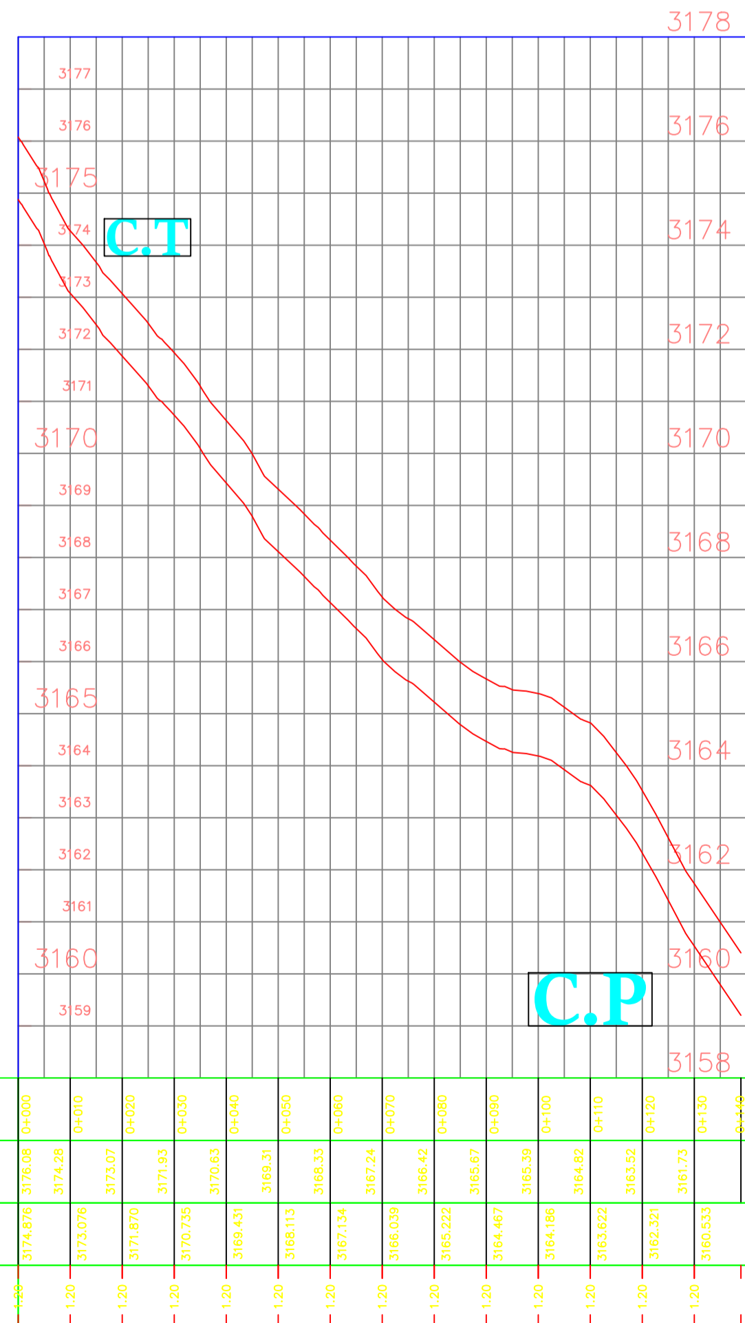
Calle 22 0+000.00 - 0+140.00
