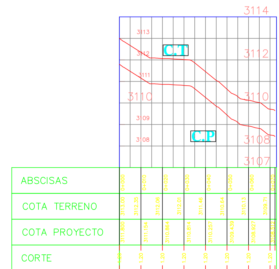
Calle 12 0+000.00 - 0+073.00
