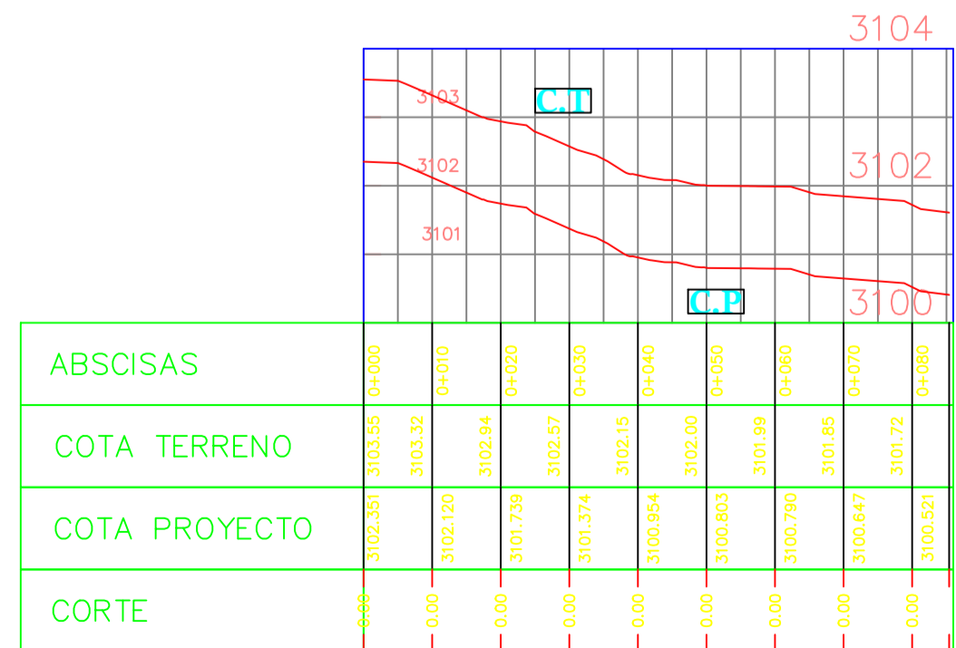
Calle 17 0+000.00 - 0+086.00
