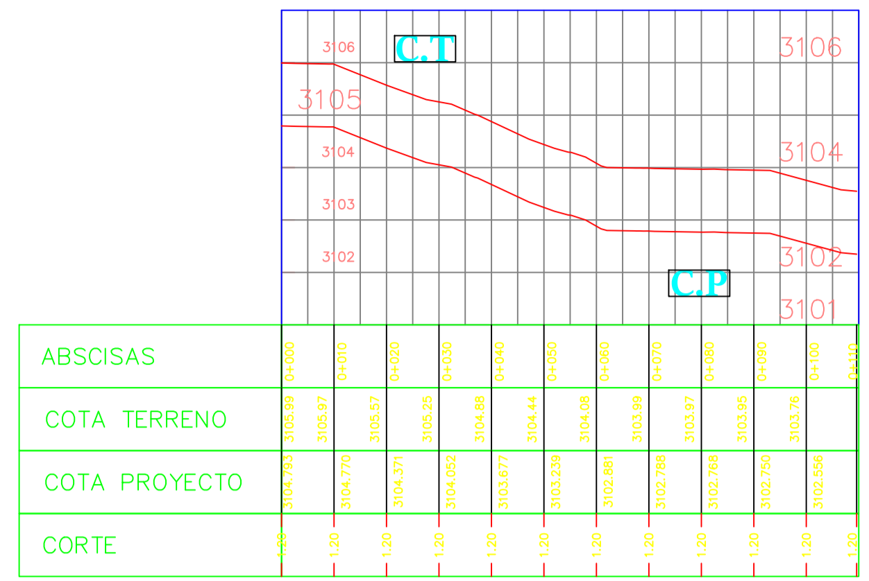
Calle 16 0+000.00 - 0+110.00
