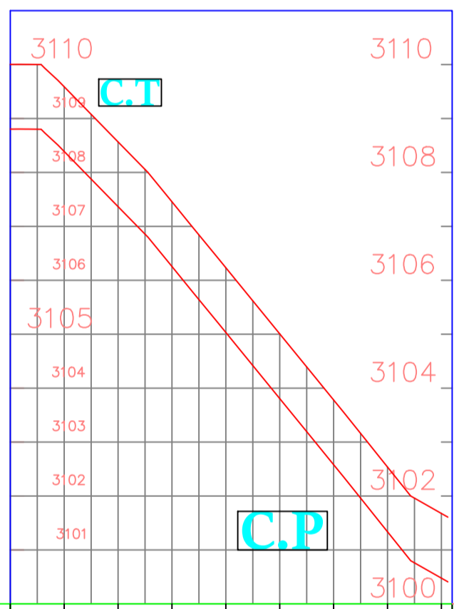
Calle 5 0+000.00 - 0+082.00
