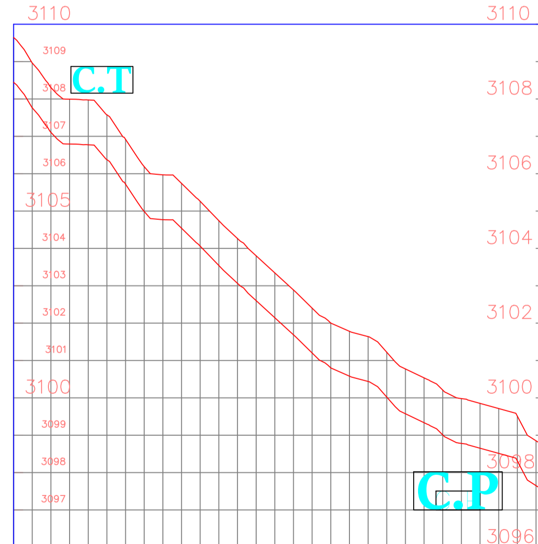
Calle 13 0+000.00 - 0+142.00
