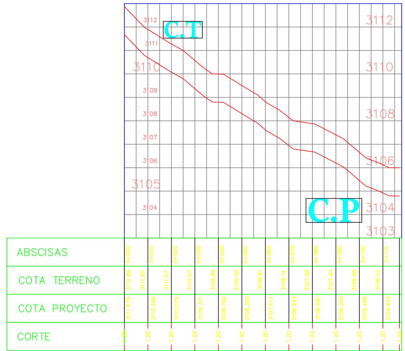
Calle 15 0+000.00 - 0+118.00
